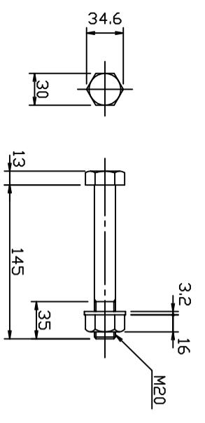
グラケット取付用B.N.W. (4,6)
